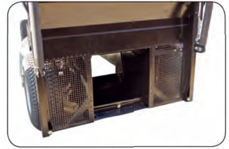
Výhozový otvor s čistící klapkou který se neucpává: Šířka odhozového tunelu je účtyhodných rozměrů 450x450 mm. Tento tunel nikdy neucpete mokrou a nebo přerostlou trávou. Patentovanou čistící klapkou vždy bezproblémově odstraníte přebytečnou trávu.
