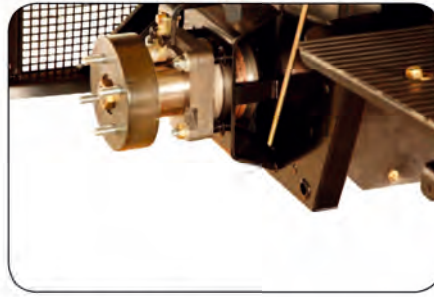
Unikátní hydropohon Pohon samostatnými kolovými hydromotory umožňuje výrazné zlepšení jízdné trakce a zároveň umožňuje zvětšení zadního výhozového tunelu pro lepší sběr trávy.
